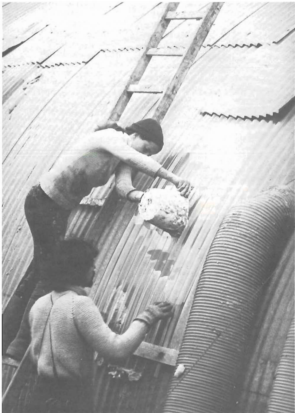
Het station wordt opnieuw geïsoleerd. Onder de oude golfplaten wordt isolatiemateriaal gegoten dat daarna uitschuimt tot ongeveer 30 \times het oorspronkelijke volume. Rechts de slurf van het hete luchtkanon waarmee de spouw op temperatuur wordt gebracht.
